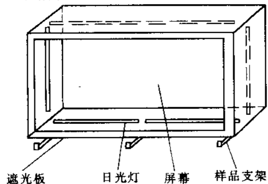
图 1 外观检验装置示意图
