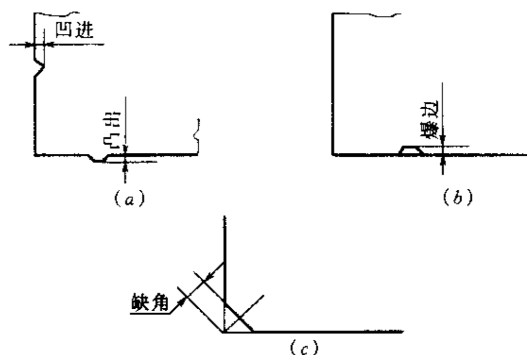
图 2 断面缺陷的测定示意图 (a) 凹凸; (b) 爆边; (c) 缺角
